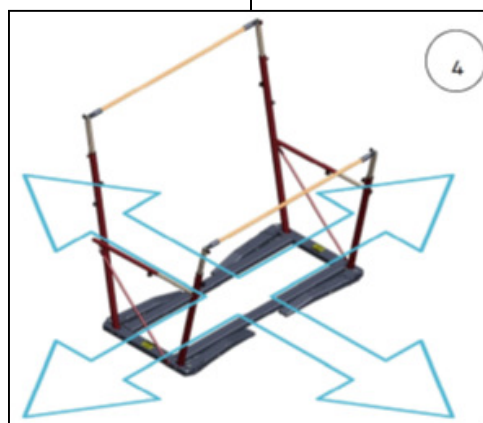
Abb. 16: 4 Bewegen des Stufenbarrens in 4 Richtungen möglich ACHTUNG! Ausleger müssen eingeklappt sein
