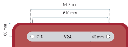
Bild 2 | Einstiegsteil Befestigung
