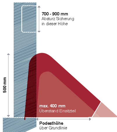
Bild 1 | Einstiegsteil
