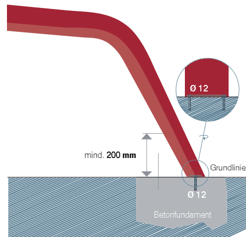
Bild 4 | Ausstiegsteil Verschraubung
