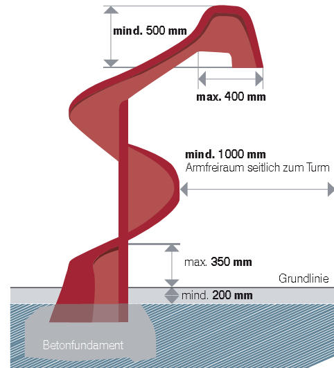
Bild 6 | Wendelrutsche
