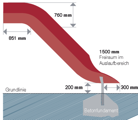
Bild 5 | Röhrenrutsche
