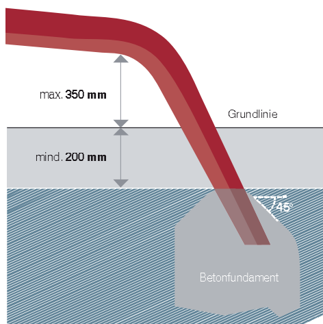
Bild 3 | Ausstiegsteil Betonfundament
