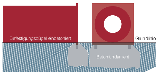
Bild 7 | Kriechröhren
