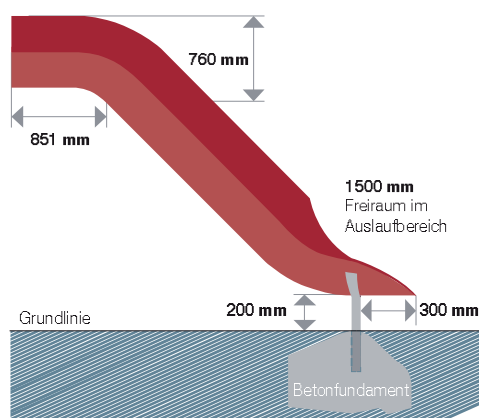
Bild 5 | Röhrenrutsche
