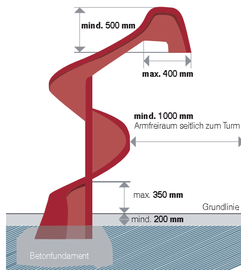
Bild 6 | Wendelrutsche
