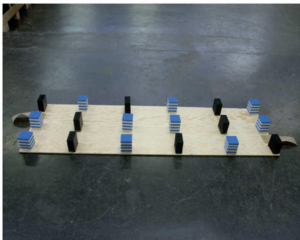
Halbe Federplatte von unten mit angetackertem Befestigungsklettband und aufgeklebten Federelementen
