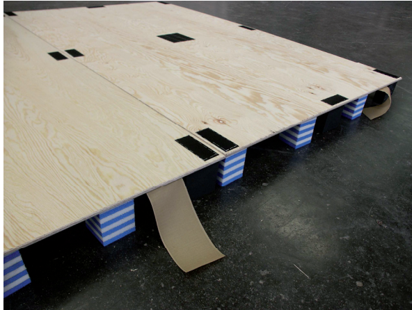
Federplatten zusammen
