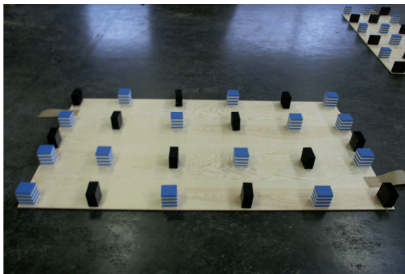
Federplatte von unten mit angetackertem Befestigungsklettband und aufgeklebten Federelementen
